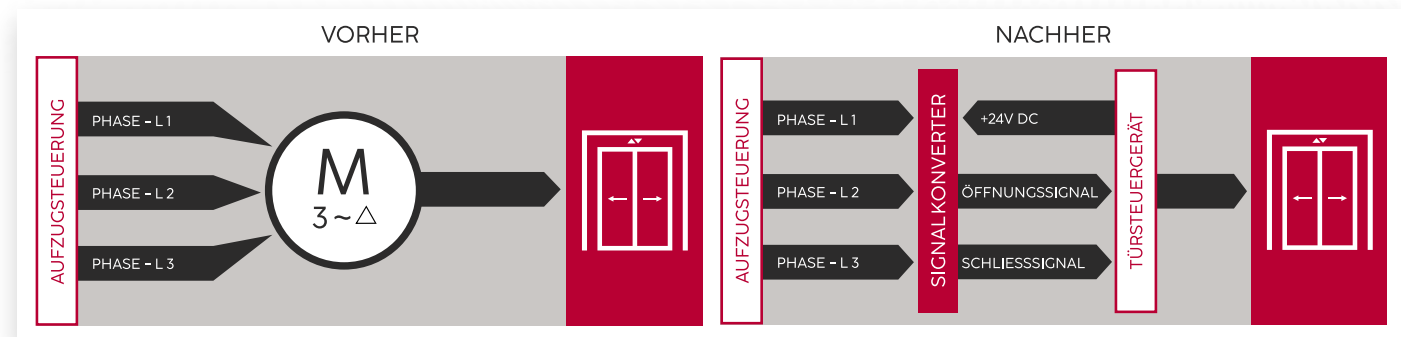
VORHER - NACHHER DARSTELLUNG DER KABINENTÜRANSTEUERUNG
